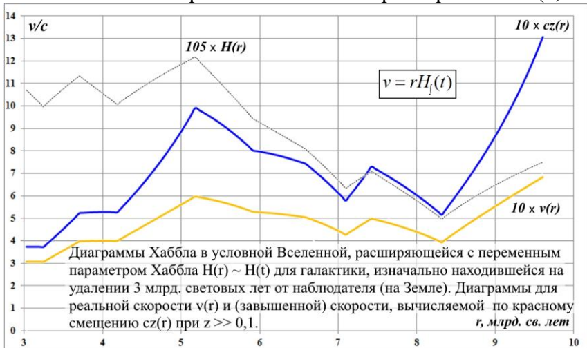
Рис.2. Диаграммы Хаббла для v(r) и cz(r) во Вселенной с параметром Хаббла H(r)
